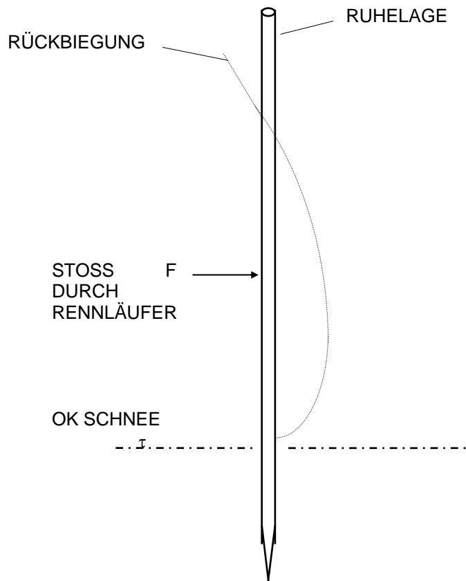
Bild 4: Definition des Peitscheneffektes
