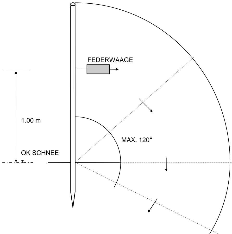
Bild 3: Definition und Prüfung des Kippwiderstandes
