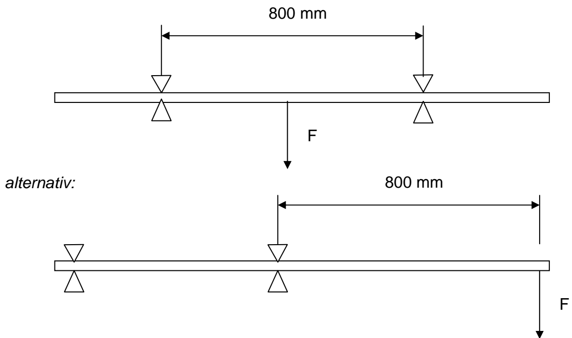
Bild 5: Einspannung für die Prüfung der Proportionalitätsgrenze im Kurzzeitbiegeversuch
