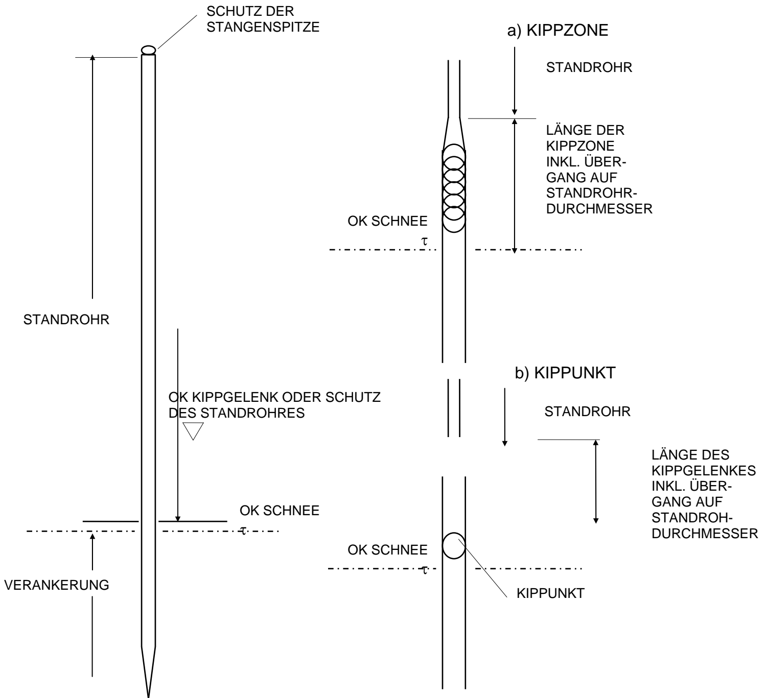
Bild 1: Definitionen zur Kippstange
