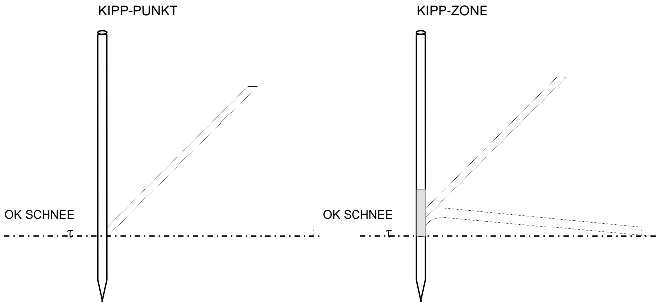
Bild 2: Funktionsweise von Kippunkt und Kippzone
